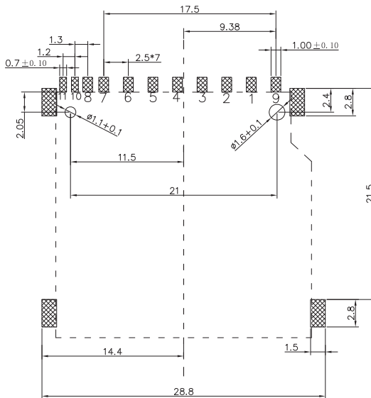
P.C.B Layout
