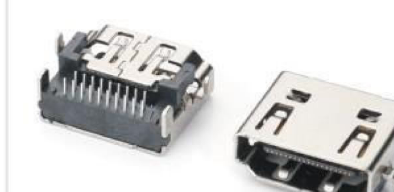
HDMI AF 正向沉板 DIP H 4.37mm
