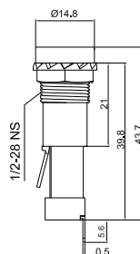
直脚 FH15-9-PZ
