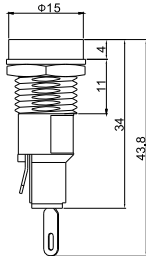
FH10-11-MZ
