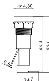
弯脚 FH15-9-PW
